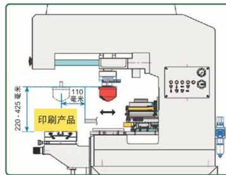
油杯平台前后推送运作 (自动清洁胶头收藏底部设计)
